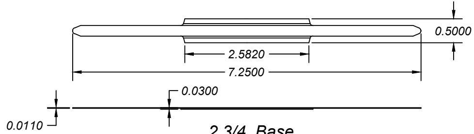
2 3/4 Base Part no:06-2B
