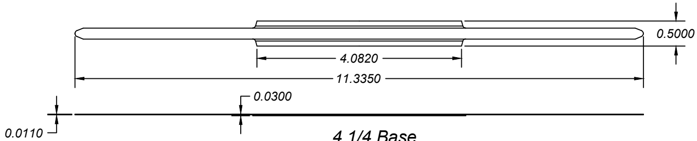
4 1/4 Base Part no:06-4B
